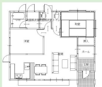
一階平面図
