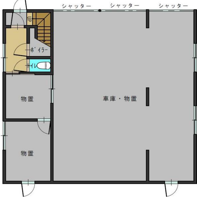
1 階
